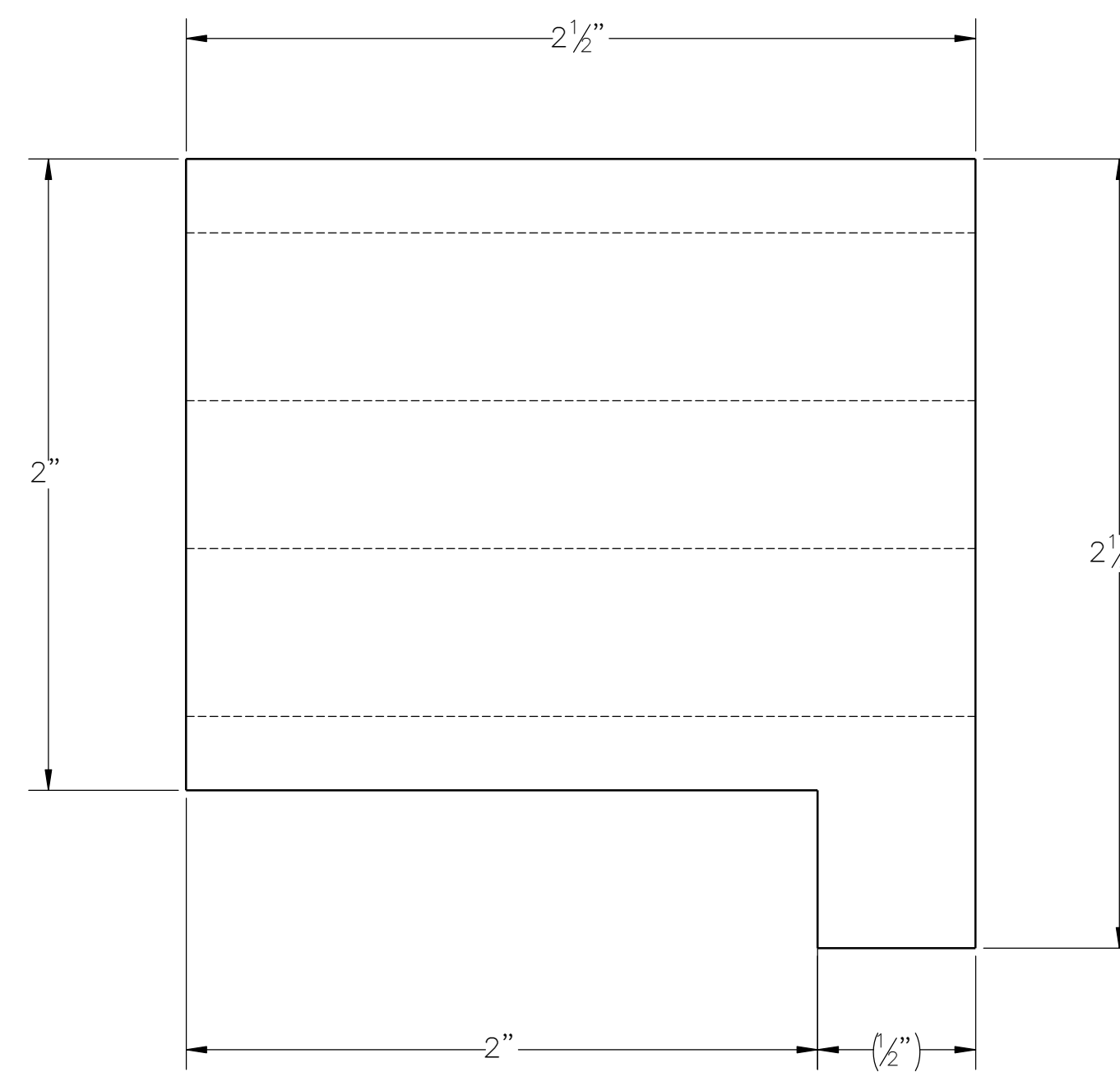
RIGHT VIEW SCALE: 2:1
