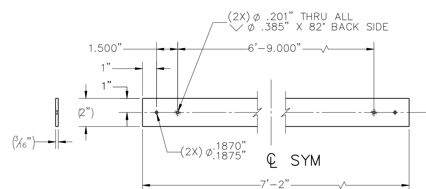
6 MIDDLE BRACE SCALE: 3" = 1'-0"
