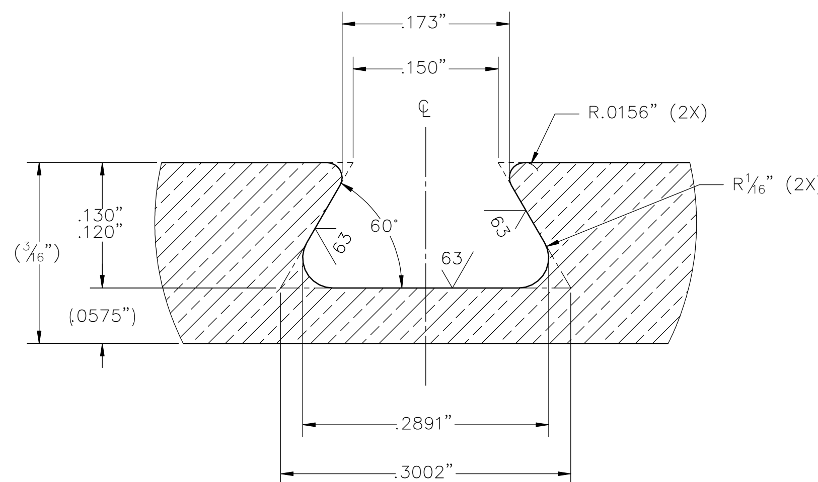
DETAIL 2 SCALE: 10:1
