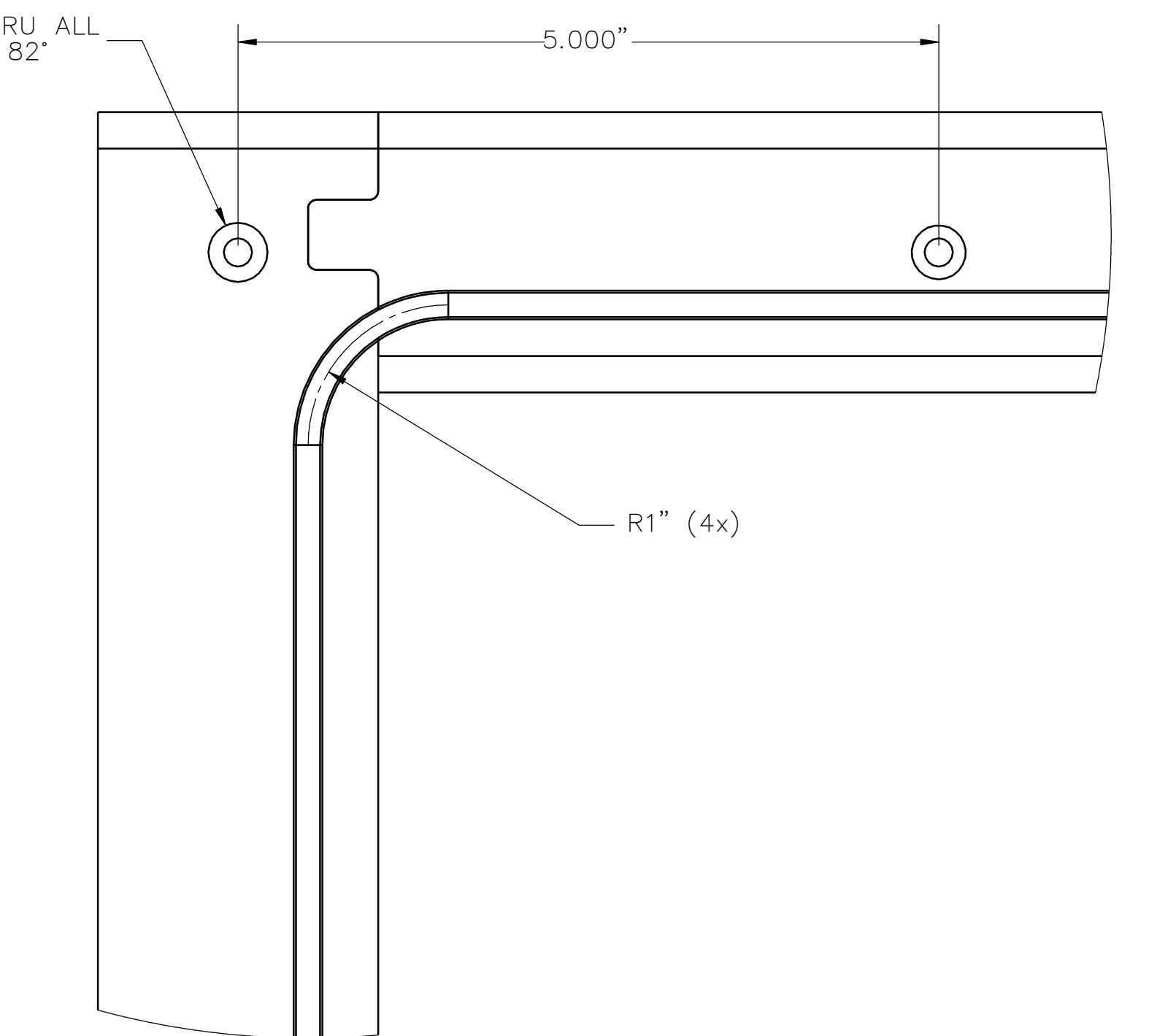
DETAIL 1 SCALE: 1:1
