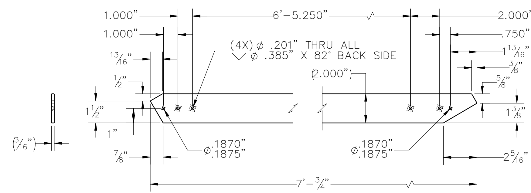
13 UPPER LEFT BRACE SCALE: 3" = 1'-0"
