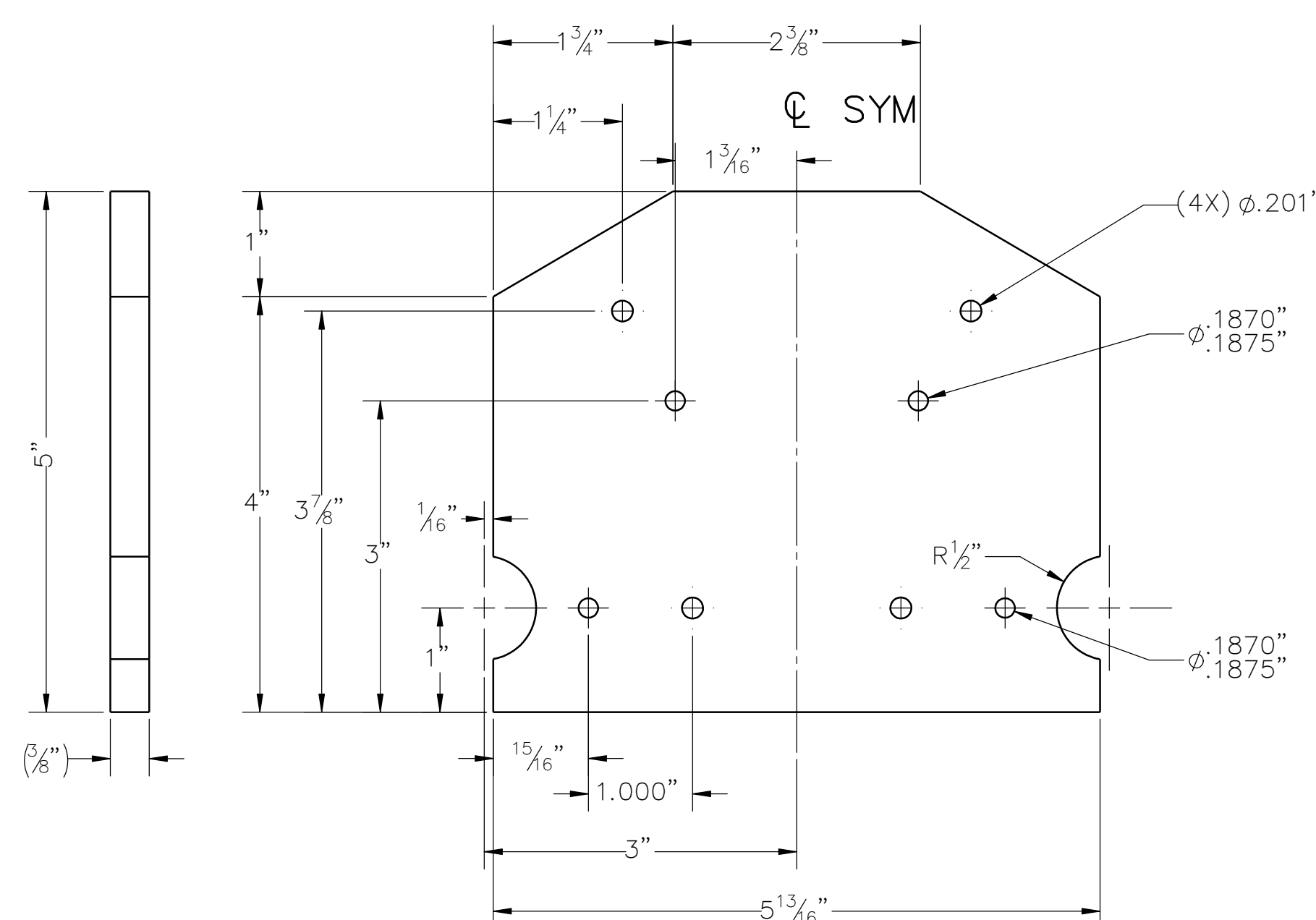
10 BOTTOM PLATE SCALE: 3/4" = 1"
