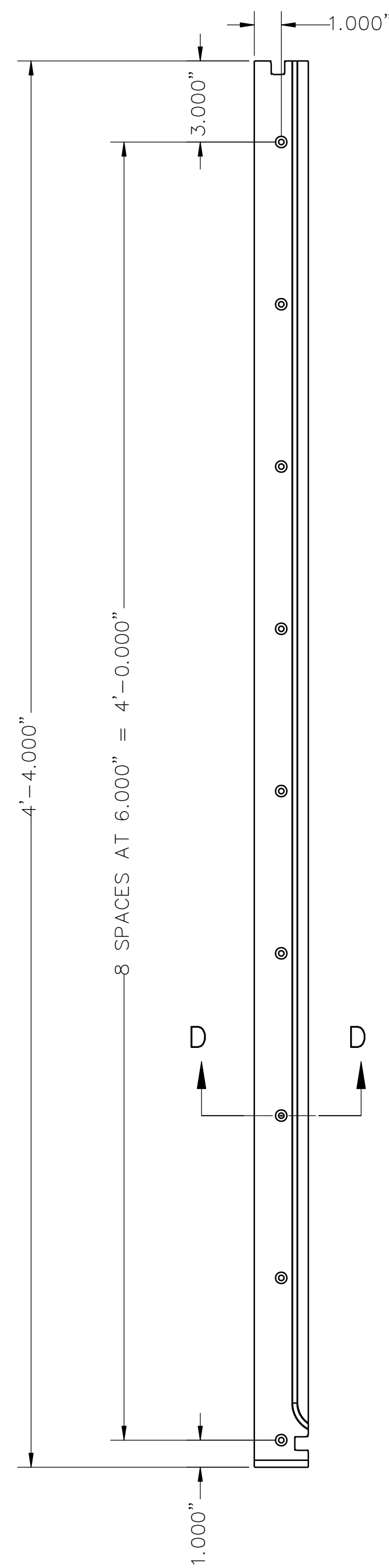
7 LOWER LEFT SCALE: 3" = 1'-0"
