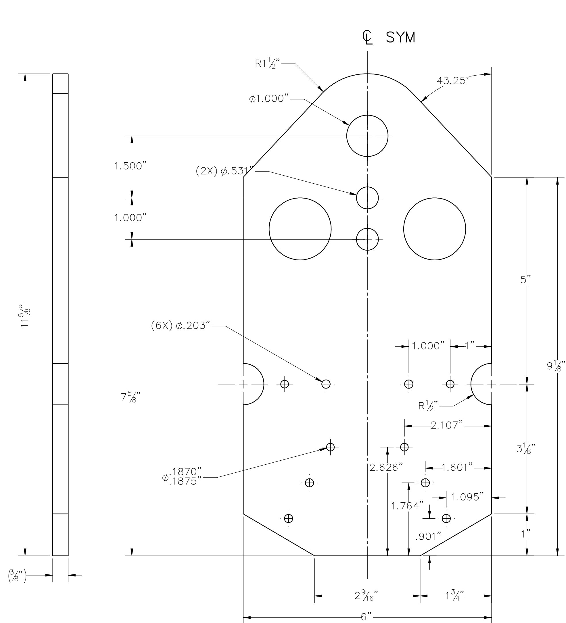
15 TOP PLATE SCALE: 3/4" = 1"
