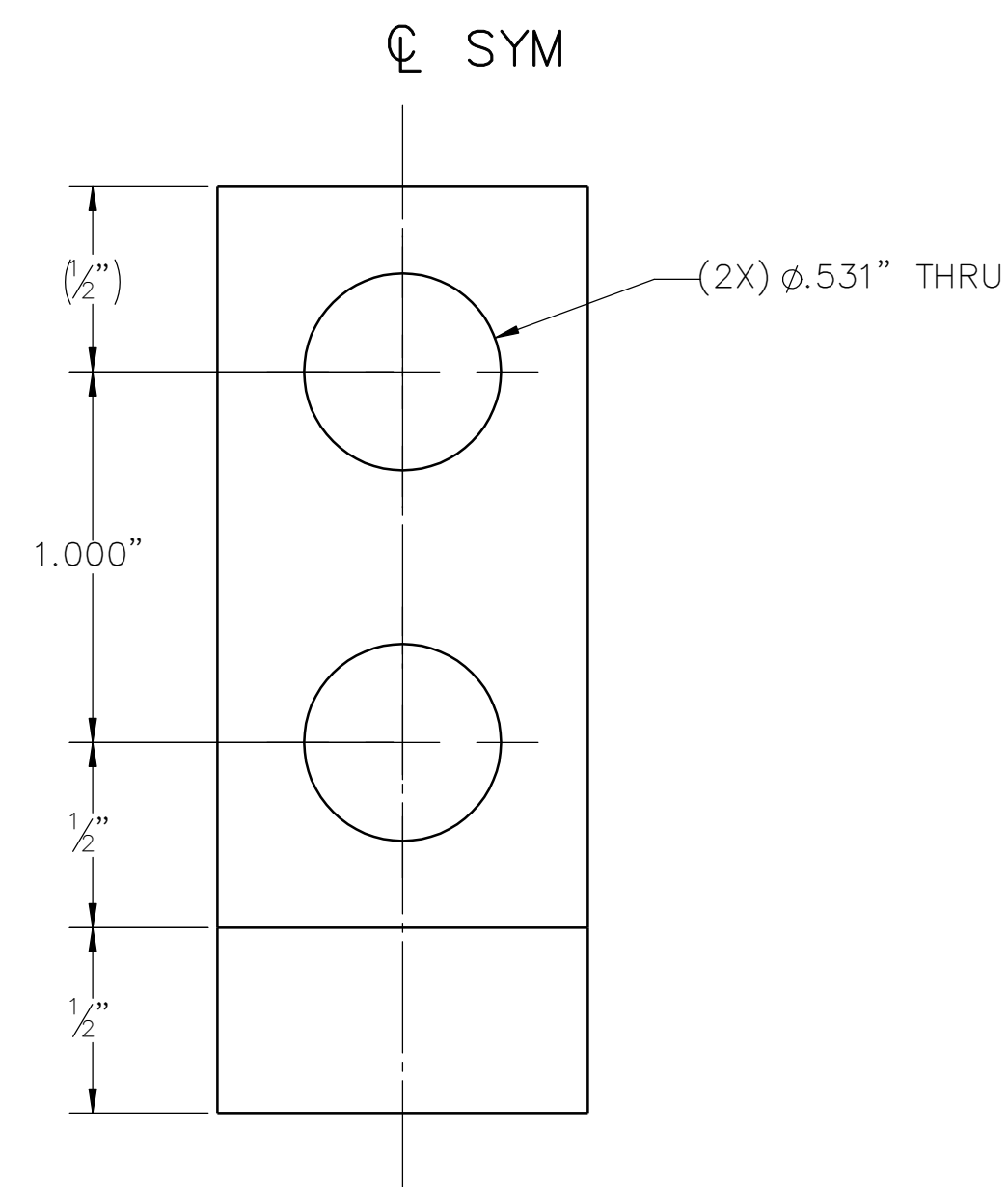
17 JIG HANGER SCALE: 2:1
