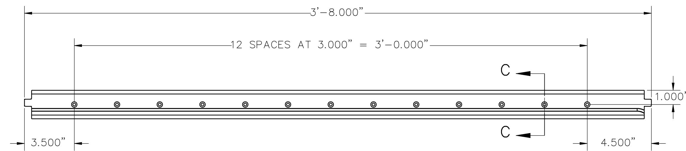
1 TOP RIGHT SCALE: 3" = 1'-0" 3
